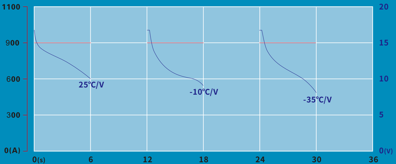
▲ TSWB-LP12V90AH在不同温度环境下的脉冲放电特性 TSWB-LP12V90AH IMPULSE DISCHARGE AT DIFFERENT TEMPERATURE
